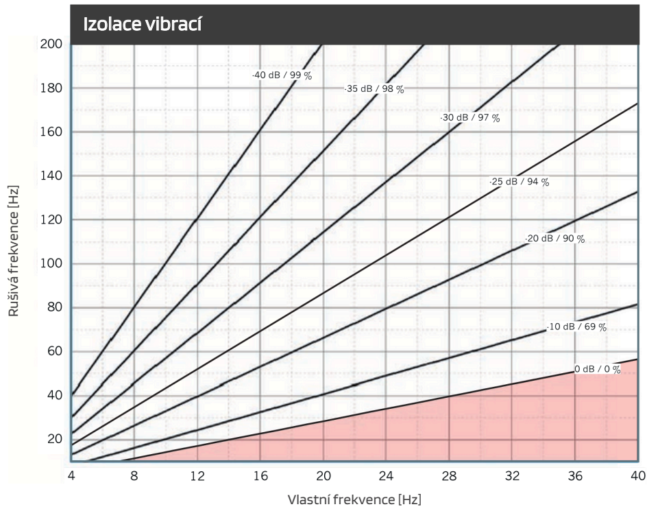
Ilustrace účinnosti izolace systému s jedním stupněm volnosti (SDOF system) na tuhém podkladu s REGUPOL vibration 450 . Parametr: přenos energie (vložený útlum) v dB, izolační činitel v %.
