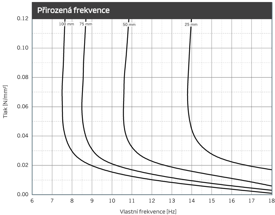
Vlastní frekvence systému s jedním stupněm volnosti (SDOF) s ohledem na dynamickou tuhost materiálu REGUPOL vibration 450 na tuhé základně. Rozměry zkušebních vzorků: 300 x 300 mm.
