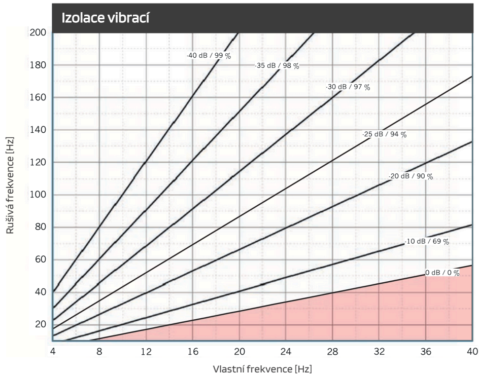
Ilustrace účinnosti izolace systému s jedním stupněm volnosti (SDOF system) na tuhém podkladu s REGUPOL vibration 300 . Parametr: přenos energie (vložený útlum) v dB, izolační činitel v %.
