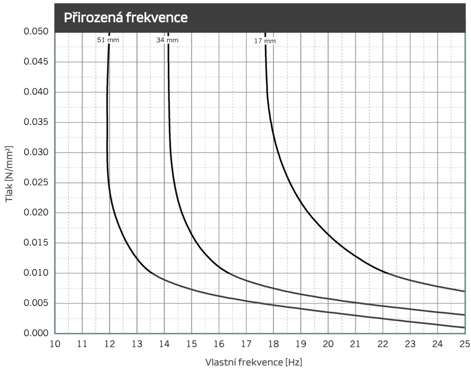
Vlastní frekvence systému s jedním stupněm volnosti (SDOF) s ohledem na dynamickou tuhost materiálu REGUPOL vibration 300 na tuhé základně. Rozměry zkušebních vzorků: 300 x 300 mm.
